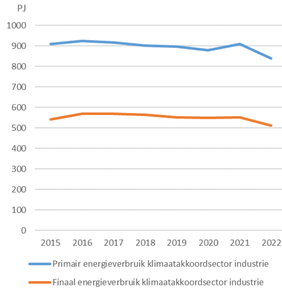
Figuur 3.7: Primair en finaal energieverbruik conform de EED in de klimaatkoördsector industrie in PJ
