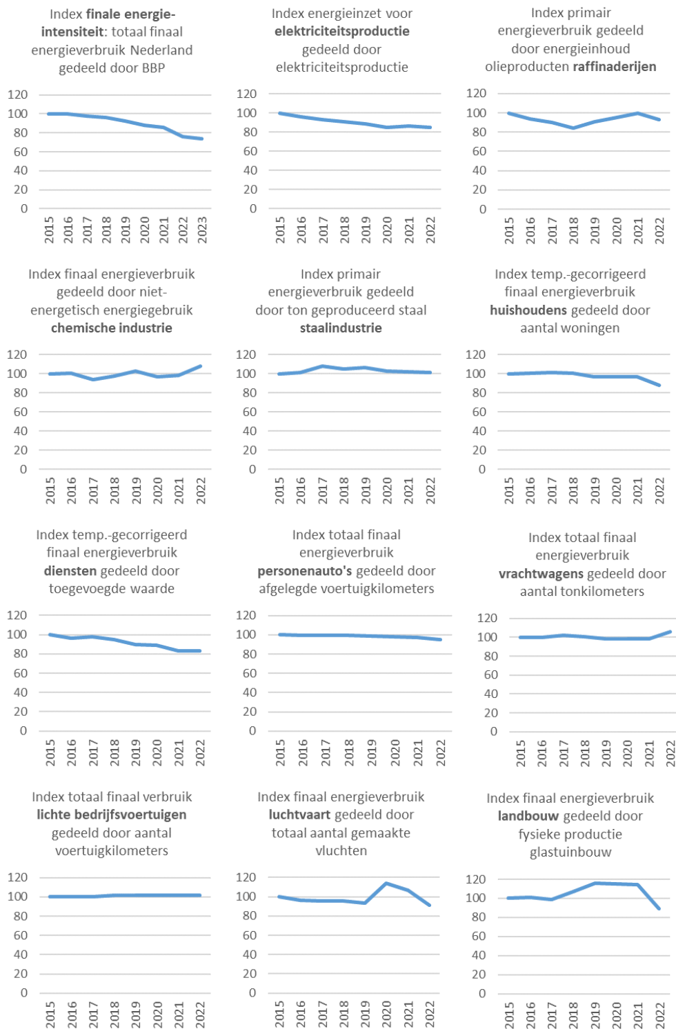
Figuur S.2: Indices voor trends in energie-intensiteit (totaal finala energieverbruik vergeleken met het BBP), energie-intensiteit van de elektriciteitsopwekking en energieverbruiken vergeleken met relevante activiteiten in de verbruikssectoren
