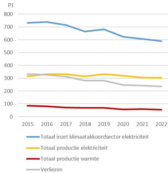
Figuur 3.4: Energie-inzet, productie van elektriciteit en warmte en verliezen in de klimaatakkoordsector elektriciteit in PJ
