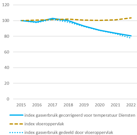
Figuur 3.19: Indices voor het voor temperatuur gecorrigeerd gasverbruik in de klimaatakkoordsector diensten, voor het vloeroppervlak en voor het gasverbruik gedeeld door het vloeroppervlak
