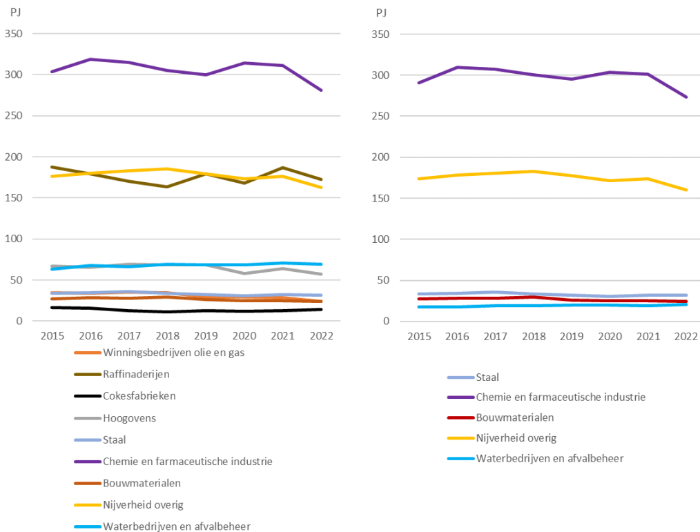
Figuur 3.10: Primair (links) en finaal (rechts) energieverbruik per subsector in de industrie in PJ
