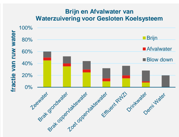
Figuur 3-13: Brijn en afvalwater afkomstig van de waterzuivering voor gesloten koelsysteem
