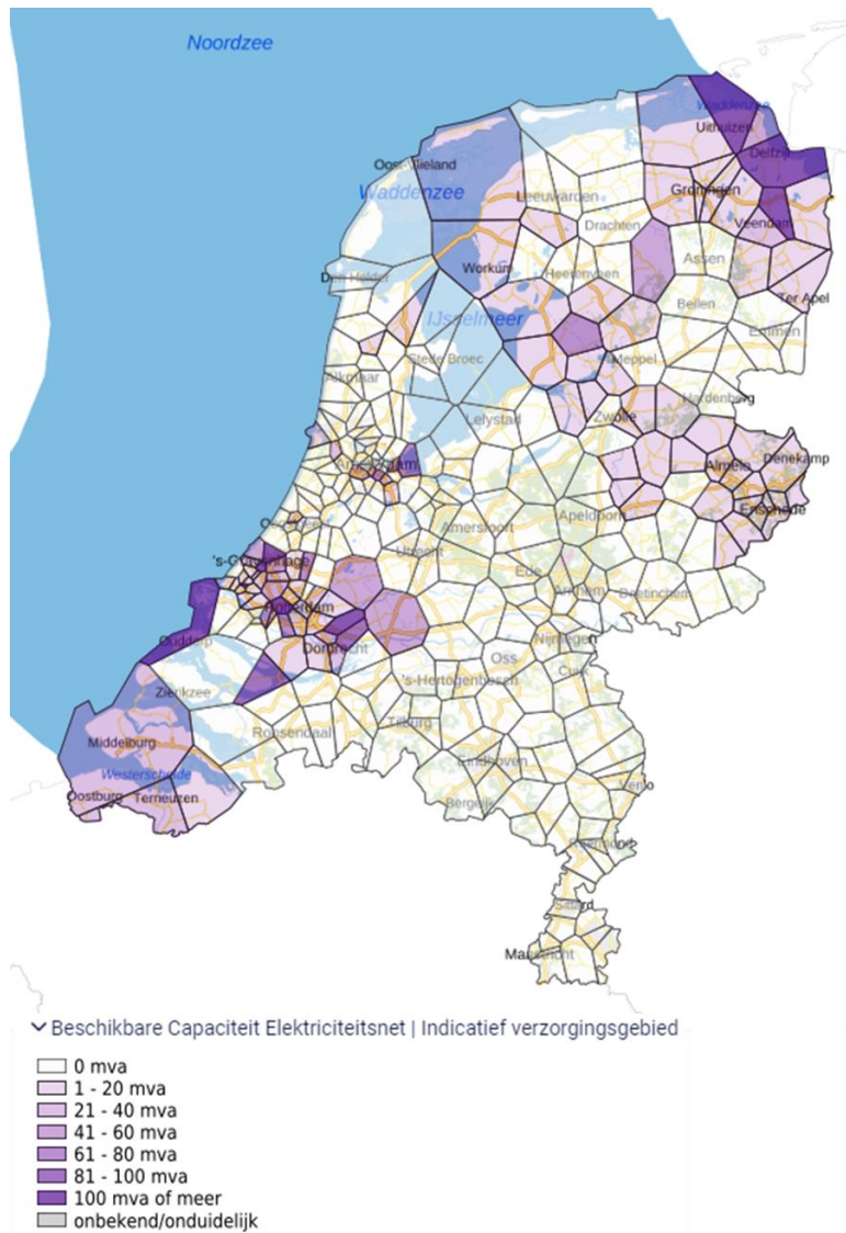
Figuur 19 - Indicatie beschikbare capaciteit op het elektriciteitsnet per provincie
