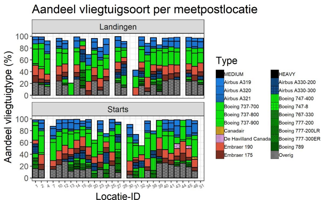
Figuur 14 Aandeel vluchtsoort per meetpost locatie, opgesplitst op basis van vliegtuigtype,
