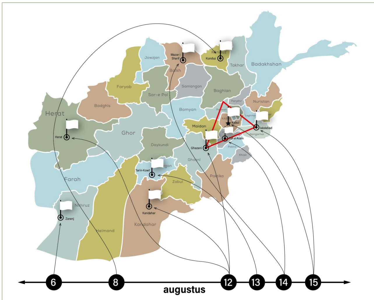
Figuur 2: Overname steden door taliban en strategische driehoek.
