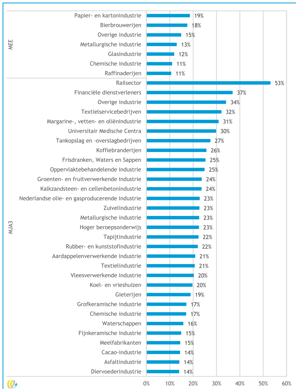
Figuur 8 - Proceefficiëntieverbetering per sector in 2020 t.o.v. 2005 in MJA3* en 2009 in MEE
