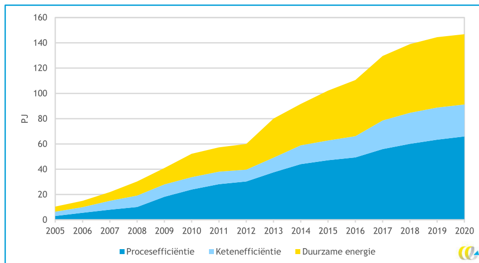
Figuur 7 - Totale cumulatieve besparingen MJA3-sectoren, 2005-2020
