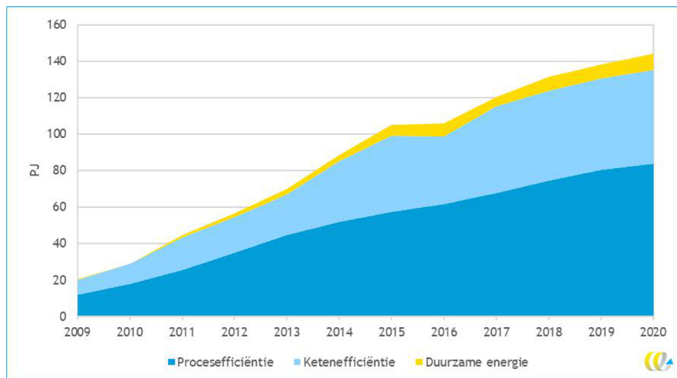
Figuur 6 - Totale cumulatieve besparingen MEE-sectoren, 2009-2020
