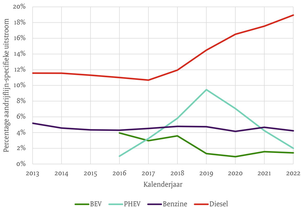
Figuur 44: De uitstroom per aandrijflijn per kalenderjaar als percentage van het aandrijflijn-specifieke wagenpark
