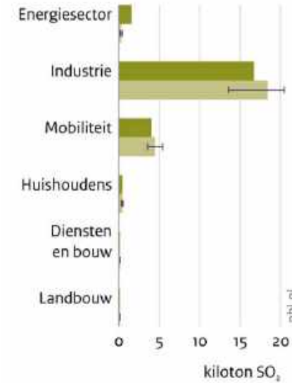
Zwavel dioxide
