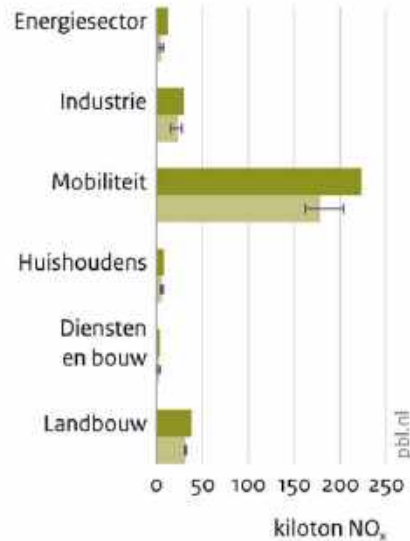
Stikstofoxiden
