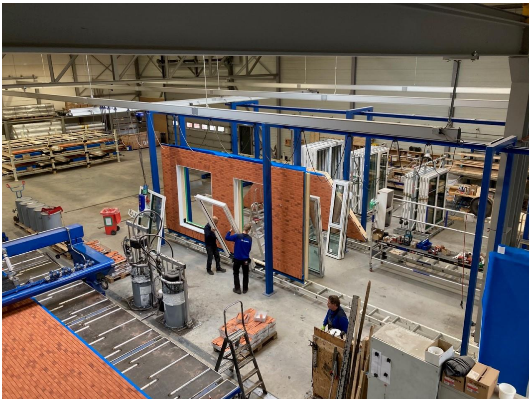
Industriële woningbouw in de fabriek van bouwgroep Dijkstra Draisma in Dokkum
