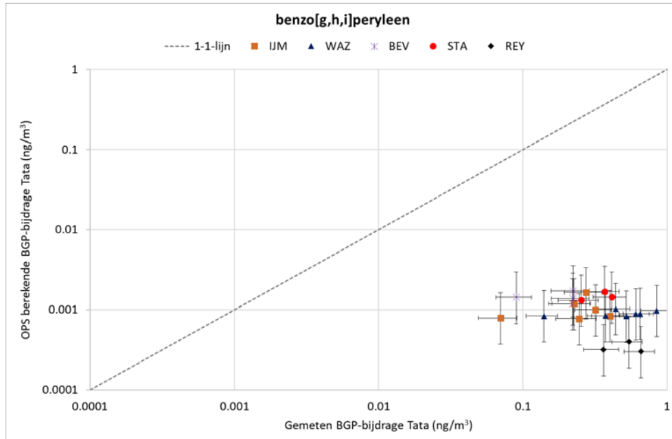
Figuur 3.13.b Berekende versus gemeten benzo[g,h,i]peryleen (BGP) concentratiebijdrage ( \text{ng}/\text{m}^3 ) door Tata Steel (2014-2020). De x- en y-as zijn logaritmisch opgemaakt
