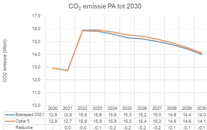
Figuur 24: CO 2 -uitstoot, optie 5.
