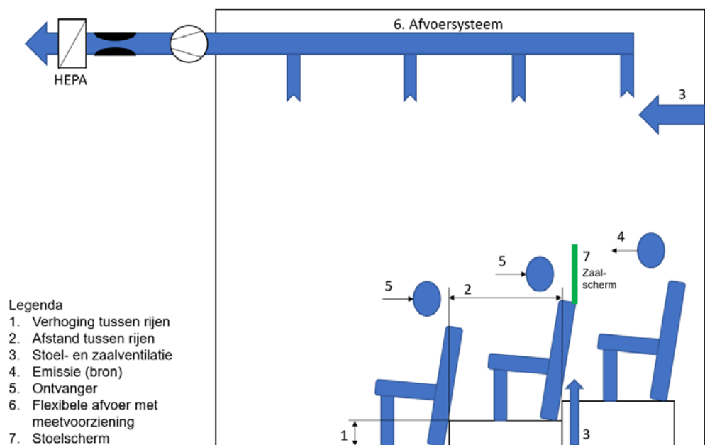
Figuur 1. Zijaanzicht mock-up meetopstelling.
