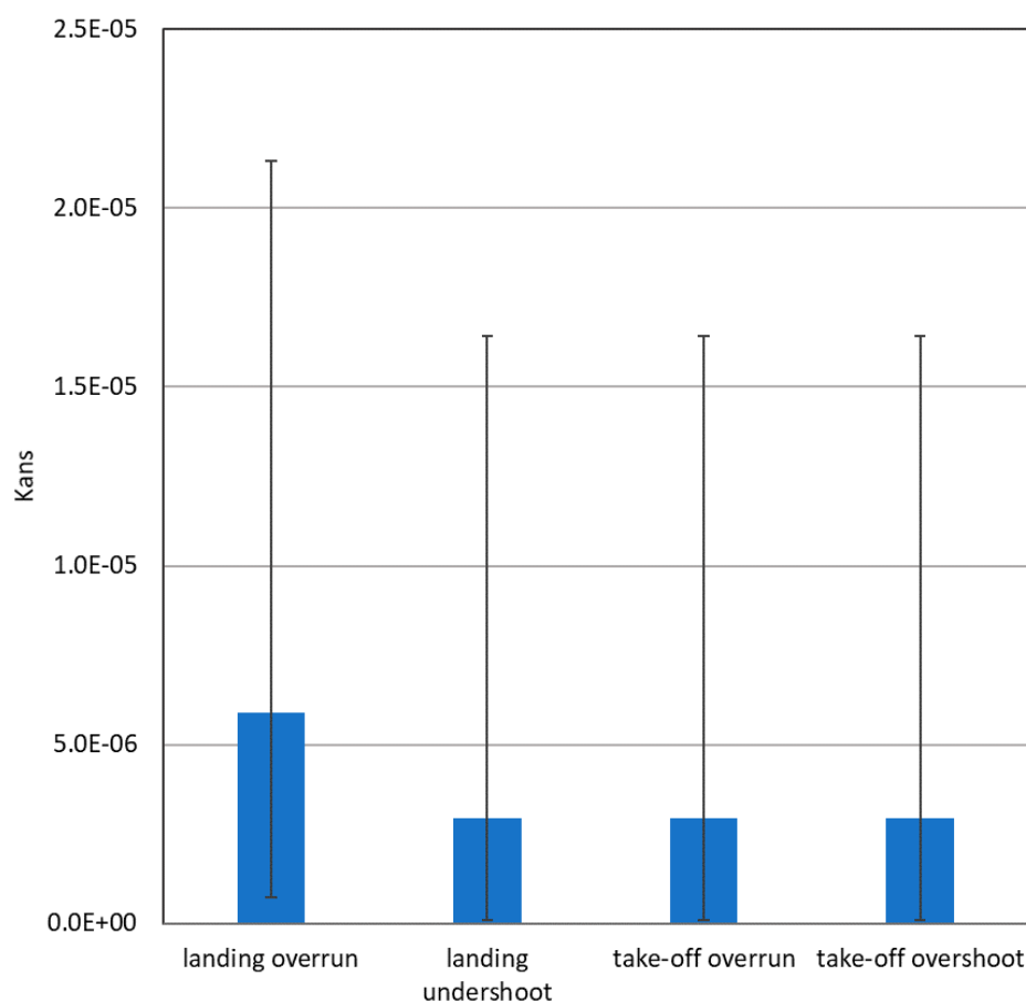
Figuur 5-3: Ongevalkansen per type ongeval voor vrachtverkeer (geregeld verkeer; periode 2005-2019) – alle generaties
