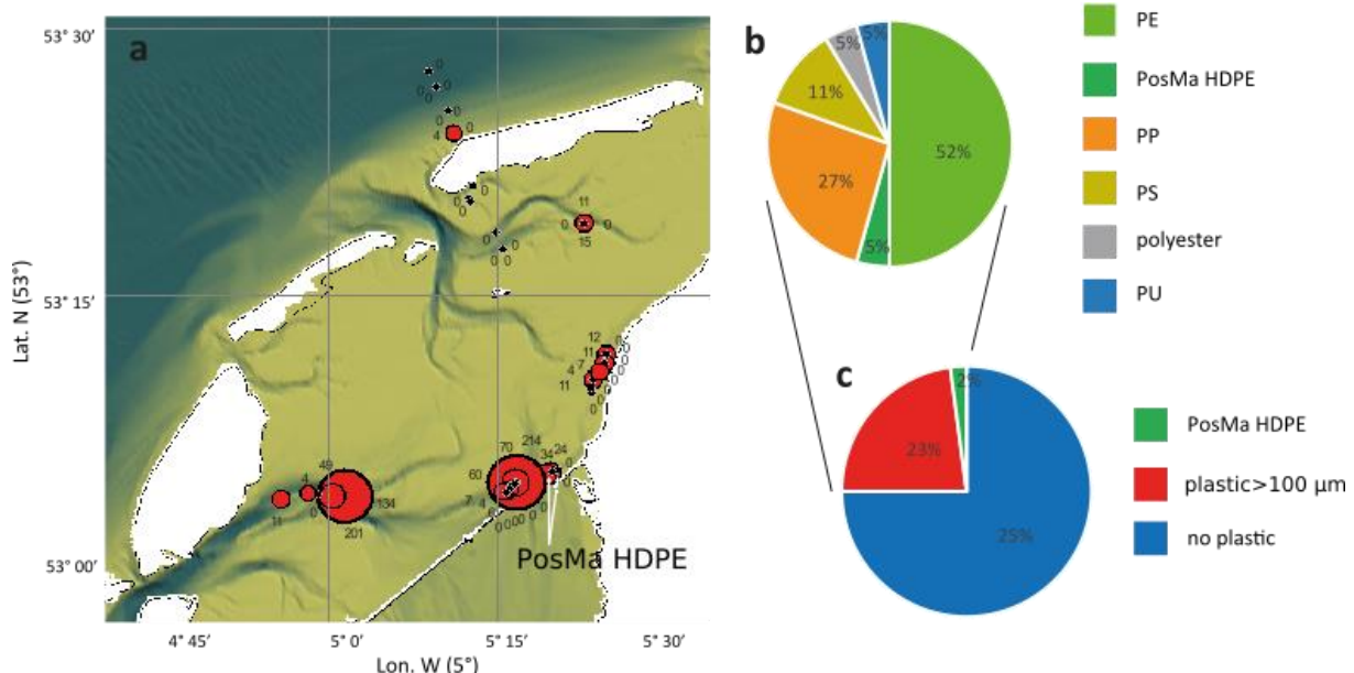
Figuur 15. Analyse van microplastics in Waddenzee water van monstercampagnes in winter, voorjaar, zomer en herfst 2019 met een neuston net (100 \mu\text{m} maaswijdte). A. De dichtheid van microplastics was zeer variabel in de ruimte, met hoogste dichtheden tot 214 plastic deeltjes per \text{km}^2 nabij de IJsselmeersluizen bij Kornwerderzand. B, C: Ongeveer een kwart van de trawls bevatte ten minste 1 deeltje plastic groter dan 300 \mu\text{m} , met PE het meest voorkomende plastic type, gevolgd door PP en PS. Er zijn 2 HDPE-pellets gevonden. PE: polyethyleen, PP: polypropyleen, PS: polystyreen, PU: polyurethaan, HDPE: hoge dichtheids polyethyleen.
