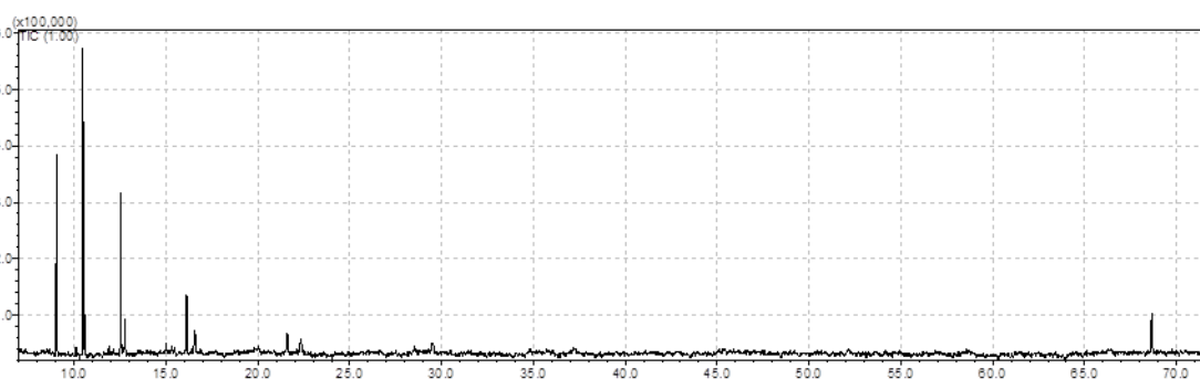
Figuur 4. GC-MS chromatogram van het geconcentreerde hexaan extract van de HDPE-pellets.
