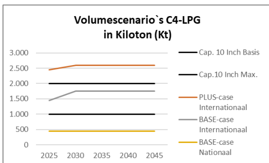
Figuur 5.2 Volumescenario's C4-LPG
