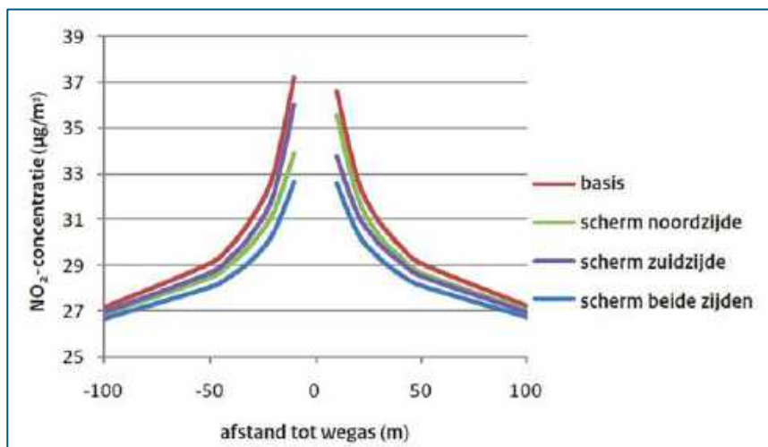
Figuur 6-2 Invloed van luchtschermen op NO 2 concentratie
