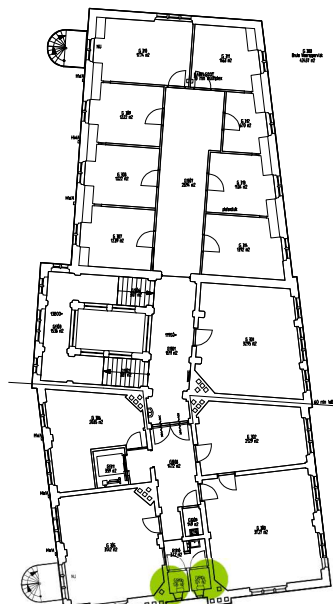
Derde verdieping
