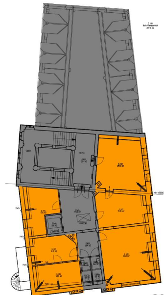
Vierde verdieping
