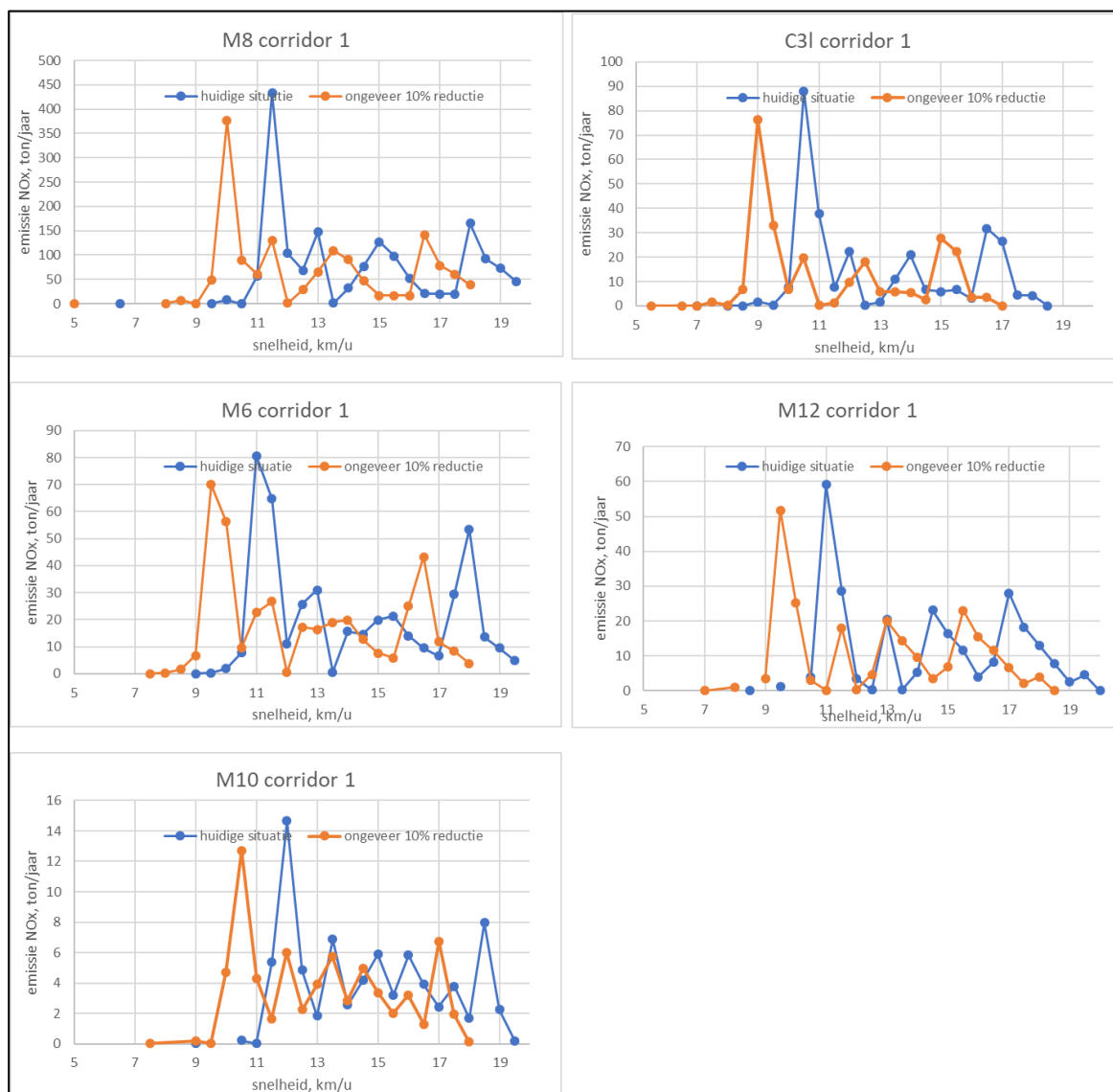
Figuur 4-3 Emissiereductie op de verbinding Rotterdam-Duitsland huidige situatie (blauw) en met snelheidsreductie (oranje).
