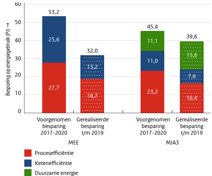
Figuur 1.2 - Voorgenomen besparing en realisatie t/m 2019 in EEP-periode 2017-2020 (MEE/MJA3)
