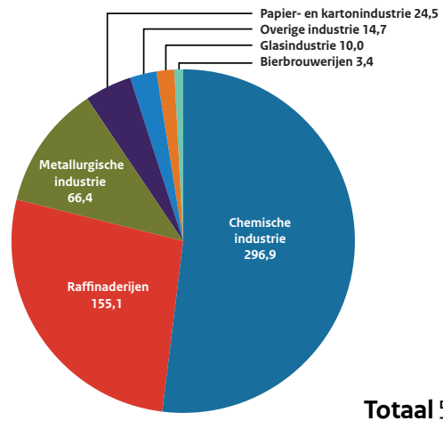
Figuur 2.1 – Primair energiegebruik per MEE-sector in 2019 (PJ)
