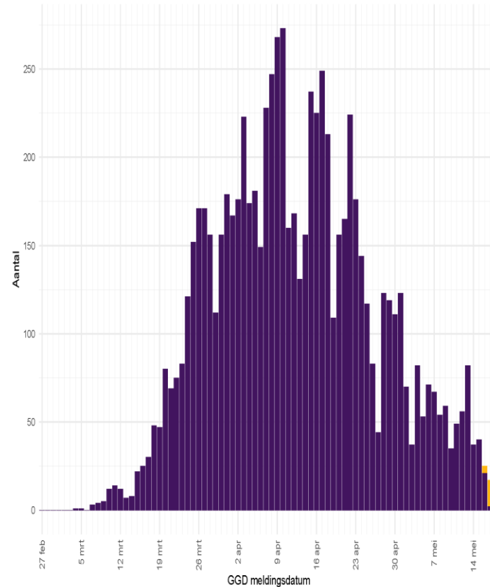
Bevestigde COVID-19+ klanten
