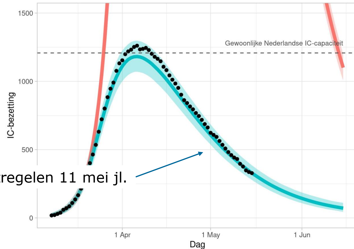
Aantal bezette IC-bedden
