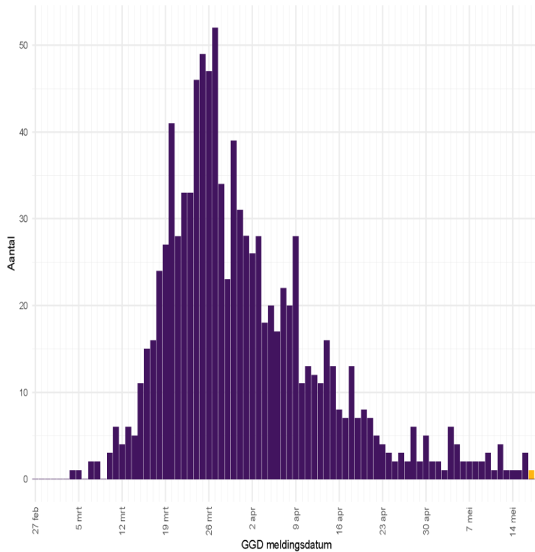
Nieuwe locaties met \geq 1 geval COVID-19
