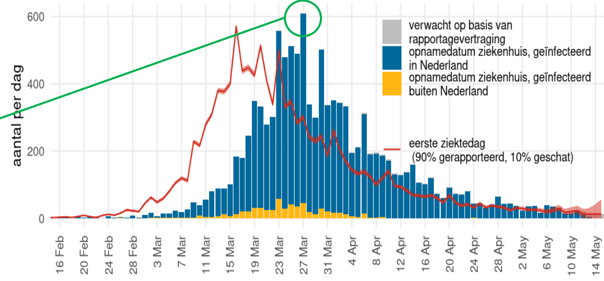
gebaseerd op ziekenhuis opnames uit OSIRIS data 2020-05-15
