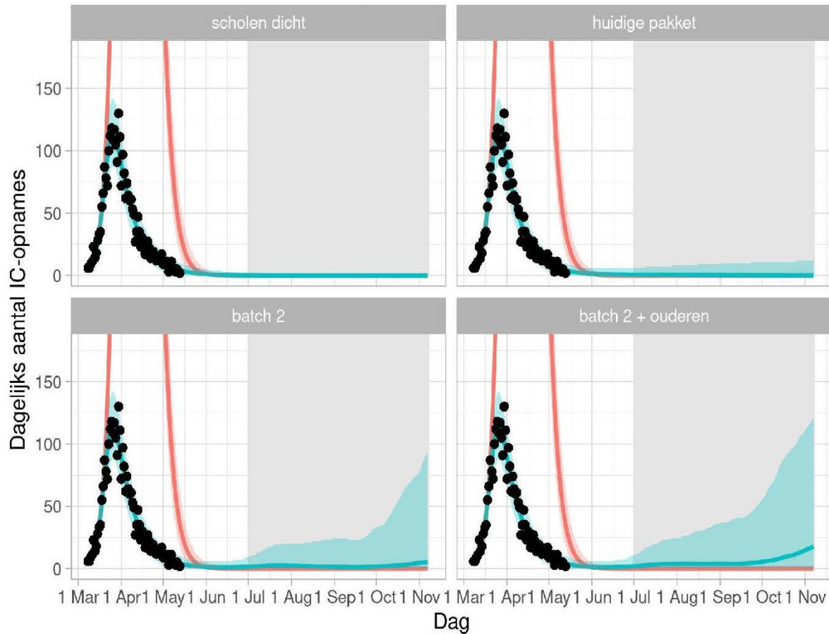
Aantal IC-opnames per dag
