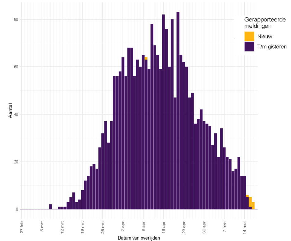
Bevestigde COVID-19+ overlijdens
