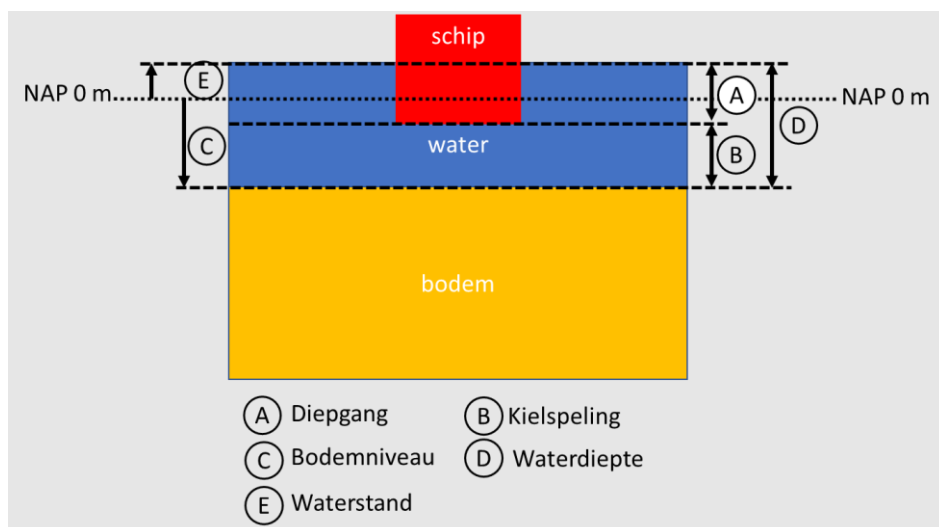
Figuur 47: Situatieschets waterstand, waterdiepte, bodemniveau, kielspeling, diepgang met bijbehorende kengetallen uit [5].
