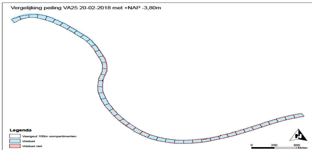
Figuur 38: Vergelijking peilingen 20-02-2018 met de vereiste bodemniveau van NAP -3,80 m in VA25
