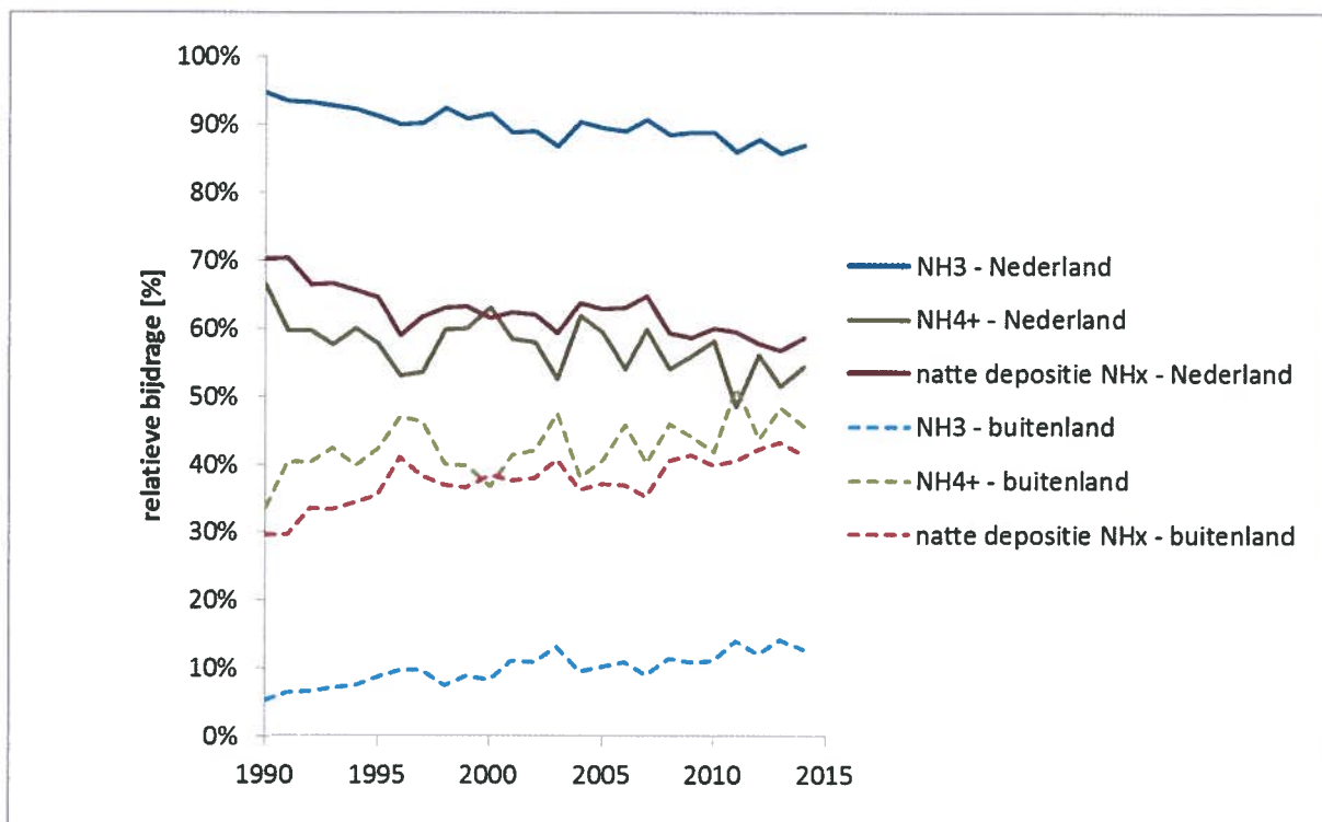
Figuur B.1. Relatieve bijdrage van Nederlandse en buitenlandse \text{NH}_3 -emissies aan de ammoniak ( \text{NH}_3 )-concentratie, de ammonium ( \text{NH}_4^+ )-concentratie in aerosol en regenwater (natte depositie).
