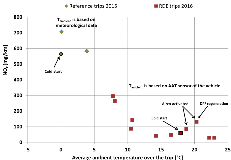
Figuur NS1 Gemiddelde \text{NO}_x -emissies van twee Mercedes C220 Euro 6 dieservoertuigen in een referentierit of RDE-rit bij verschillende omgevingstemperaturen. Meetdata zijn 'ruwe' meetdata, d.w.z. deze zijn niet genormaliseerd met de voor RDE ontwikkelde tools EMROAD en CLEAR.
