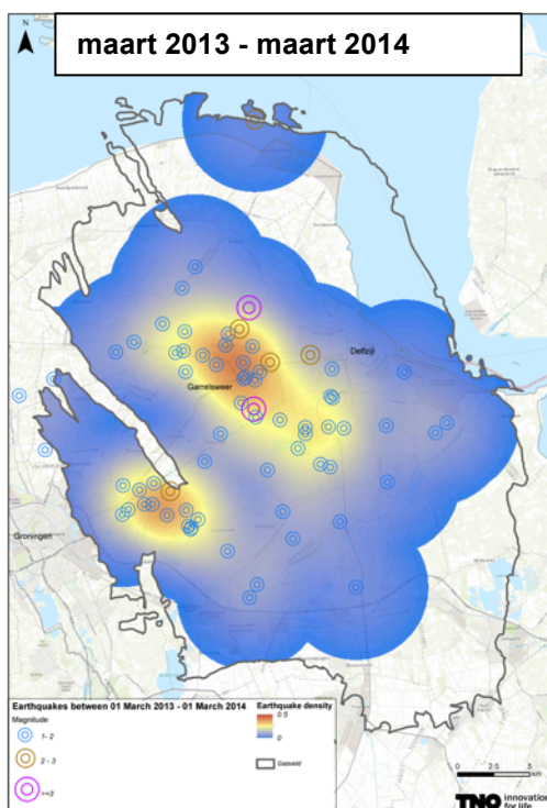
Aardbevingsdichtheid van opgetreden bevingen ( M \geq 1,0 ) voor twee verschillende perioden. Oranje betekent een relatief hoge dichtheid, blauw een lage. Gedurende het laatste jaar is de dichtheid overal lager dan twee jaar geleden.
