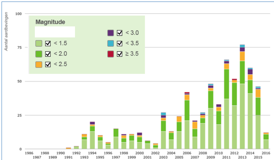
Aantal bevingen met een magnitudo van 1,0 of hoger per jaar voor het hele Groningeveld (2016 t/m 31 mei)
