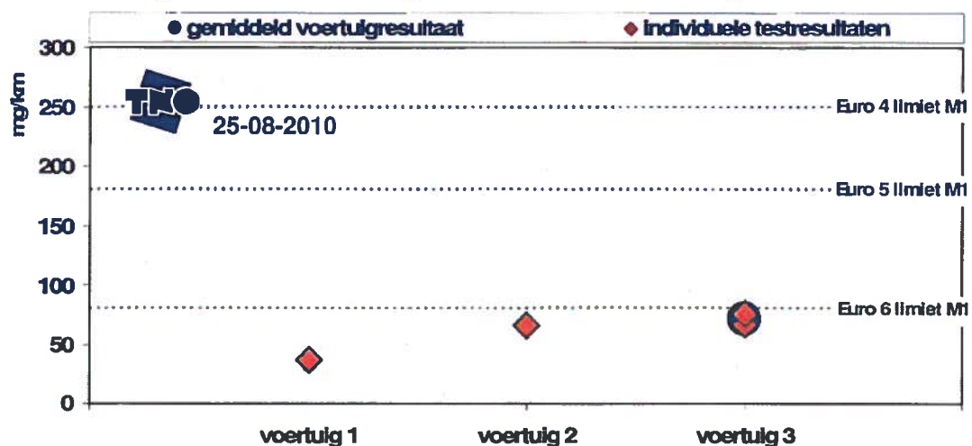
Figuur 5: \text{NO}_x -emissie tijdens de typekeurcyclus
