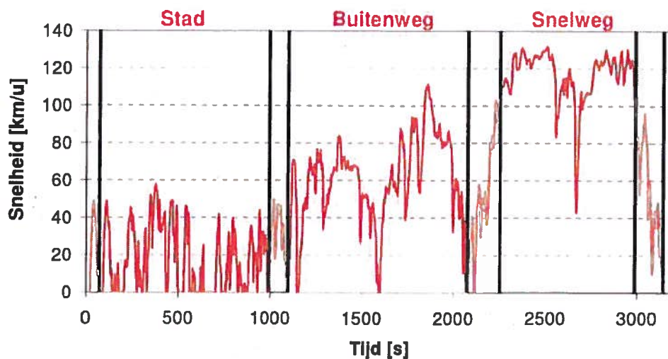
Figuur 4: CADC ritcyclus, representatief voor gemiddeld Europees praktijkgebruik van personenwagens
