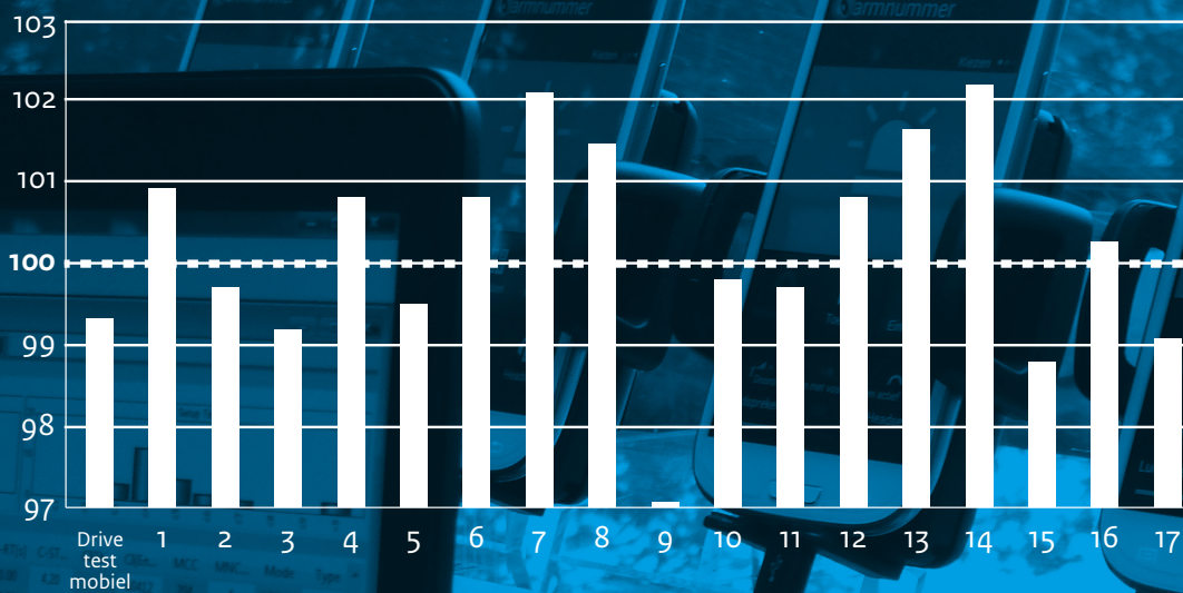
Relatieve gevoeligheid van de telefoons ten opzichte van het gemiddelde gevoeligheidsniveau (stippellijn) van alle geteste toestellen
