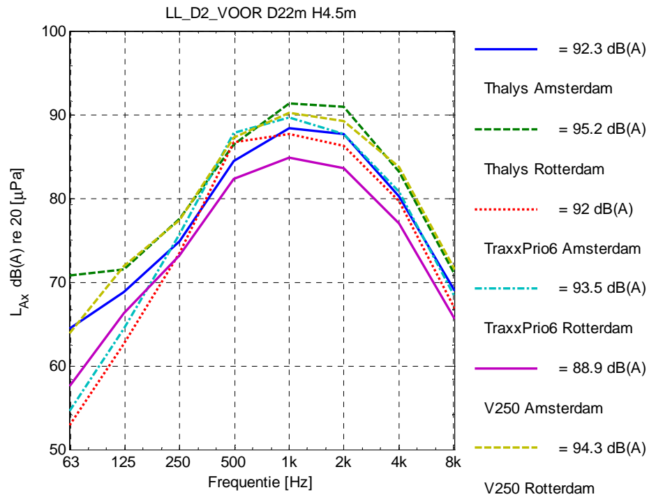
Figuur 16 Gemiddelde octaafspectra van het geluidexpositieniveau bij meetdoorsnede 2, Thalys, V250 en TraxxPrio in beide richtingen.
