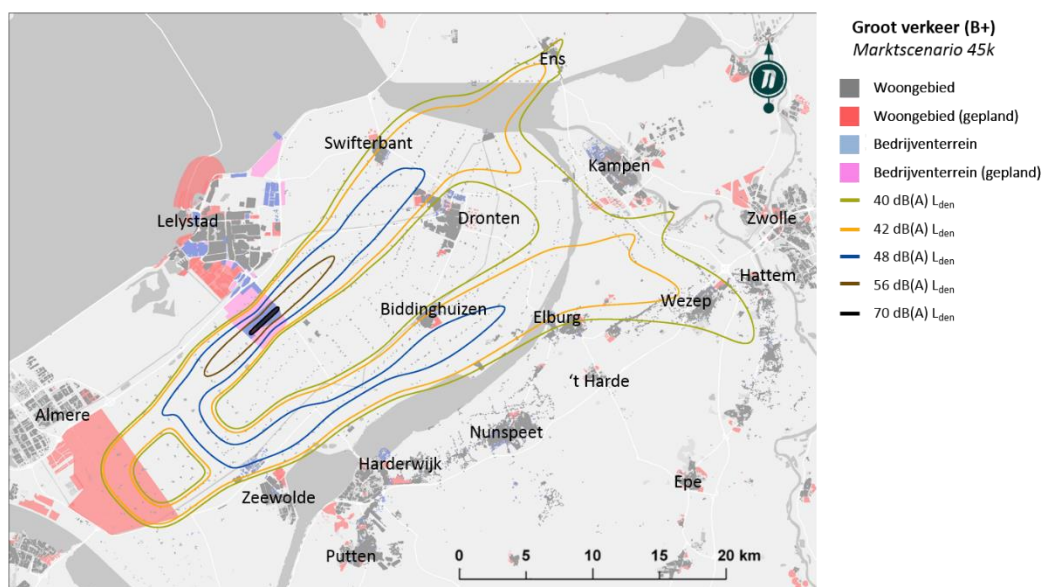
Figuur 38 - Geluidscontouren voor alleen het groot verkeer bij 45 k voor B+
