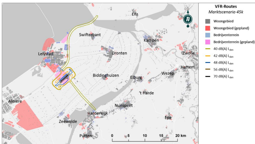
Figuur 37 – Geluidscontouren voor alleen het klein verkeer bij 45 k.
