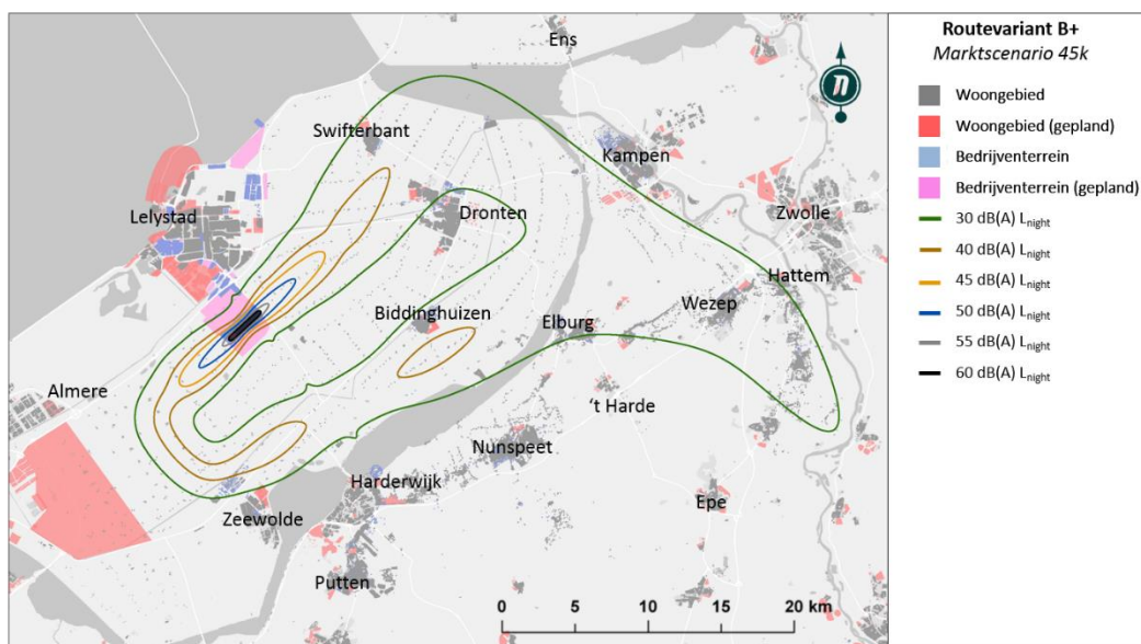
Figuur 46 – Geluidscontouren L_{night} Variant B+ 45k marktscenario
