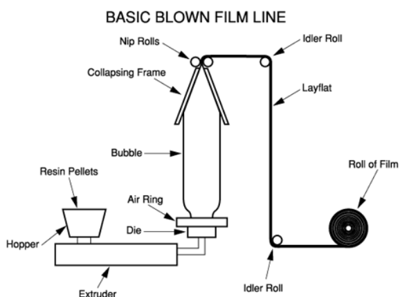
Figuur 2.5 Proces van folieblazen [Plasticstech, 2014].
