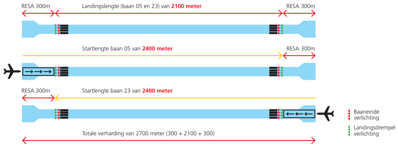
Figuur 6.4 Beschikbare baanlengte Lelystad Airport
