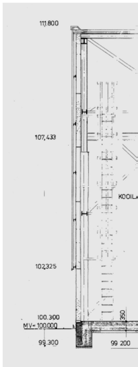
Figuur 6.19 Constructie gebouw (tekening A-409-CG-218) waar de leiding aan zit bevestigd
