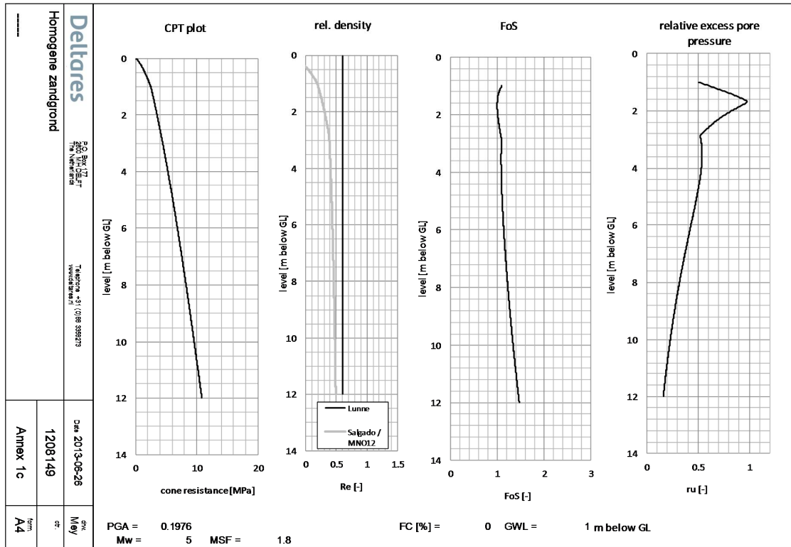
Figuur 6.5 Voorbeeld berekening verweking
