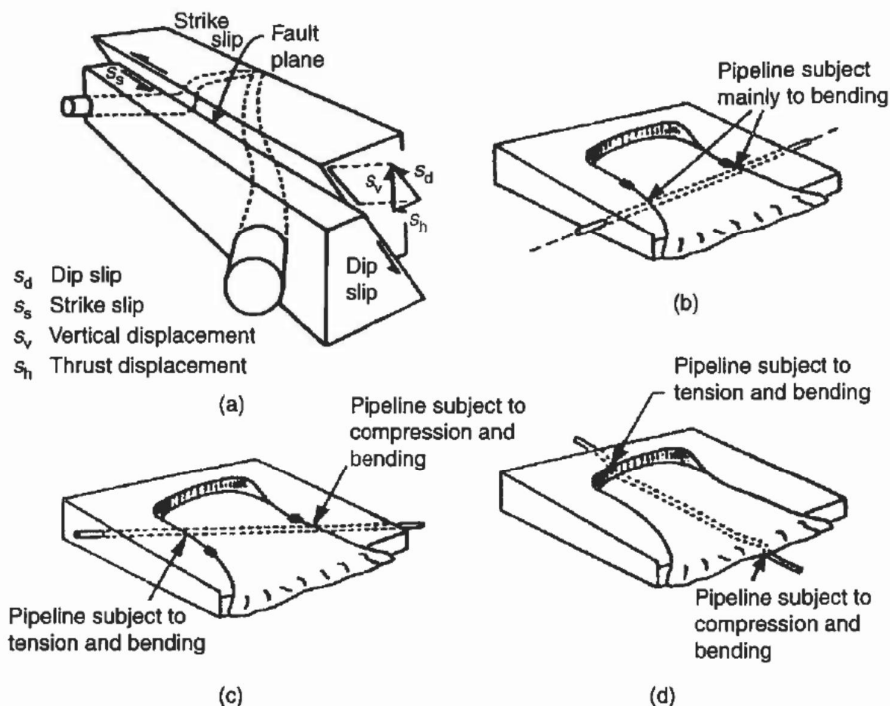
Figuur 5.2 Permanente grondbewegingen (O'Rourke et al 2001)
