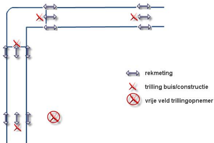
Figuur 7.1 Bovenaanzicht haakse bocht (schematisch weergave)
