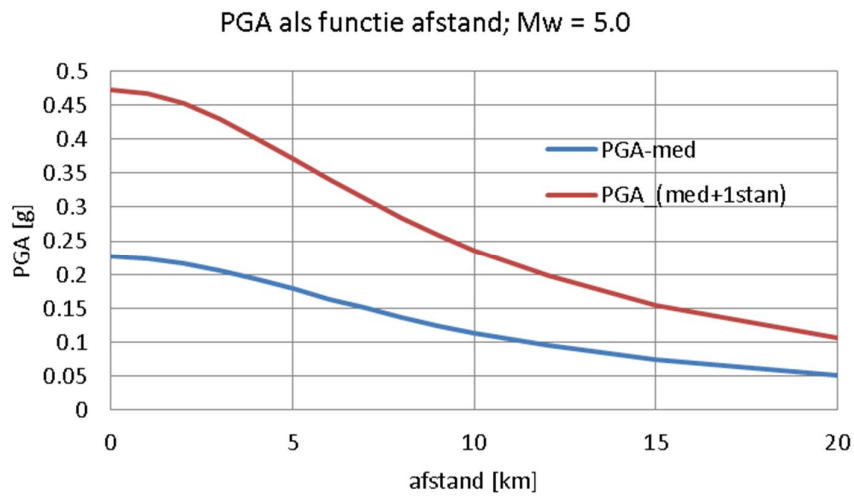
Figuur 4.3 PGA als functie afstand, Mw = 5
