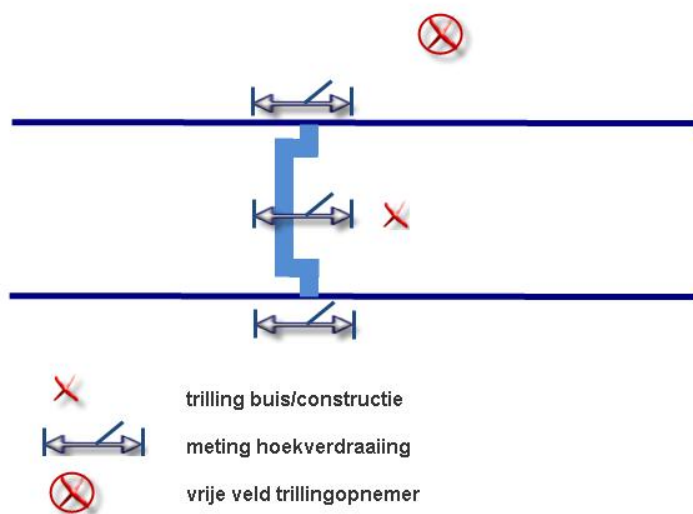
Figuur 7.3 Bovenaanzicht schematische doorsnede isolatiekoppeling
