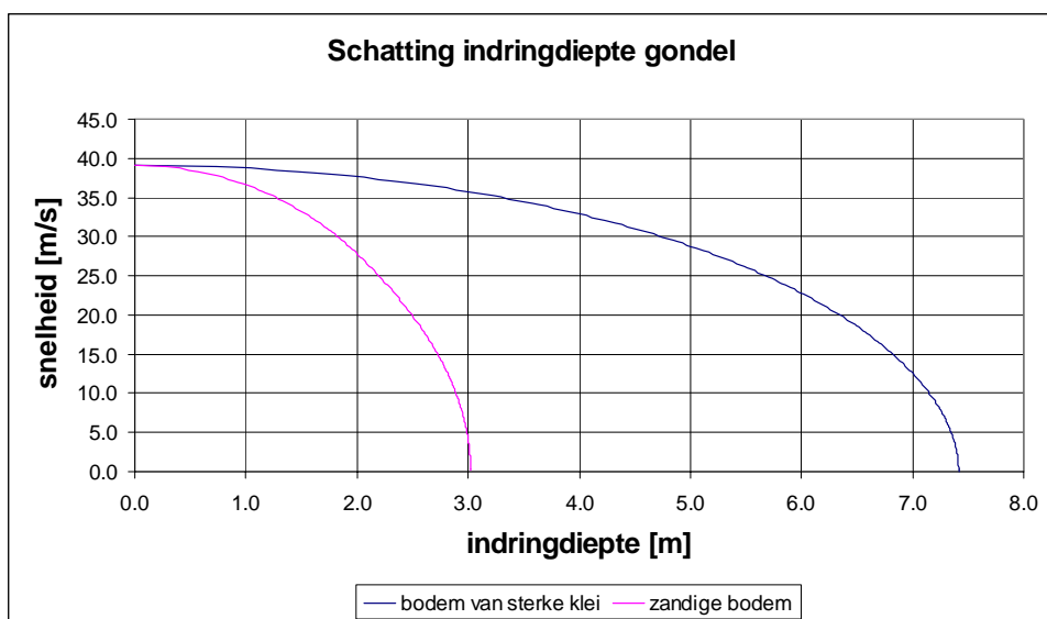
Figuur 6.35 Berekening van de indringingsdiepte van een vallende gondel van een windmolen
