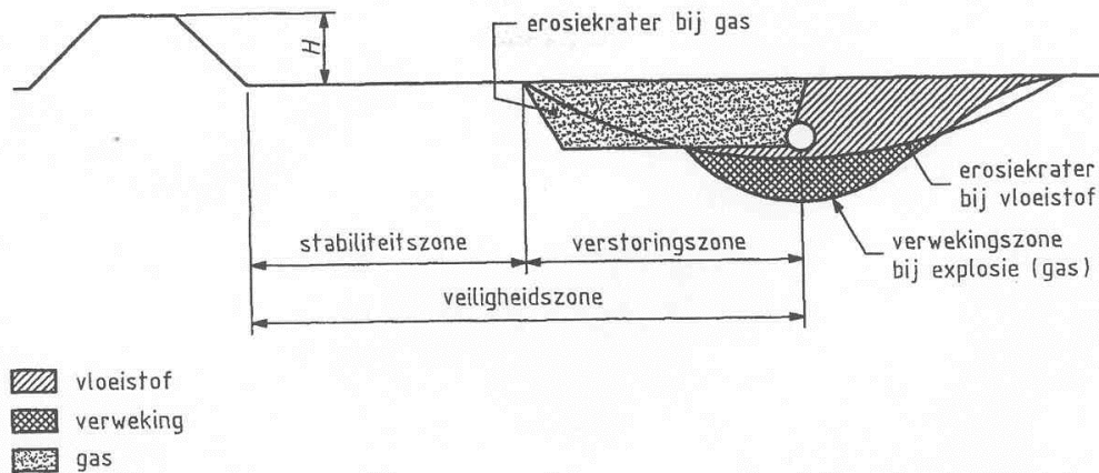
Figuur 6.34 NEN 3651 stabiliteitszone van de waterkering en de voorgeschreven ligging van een gasleiding
