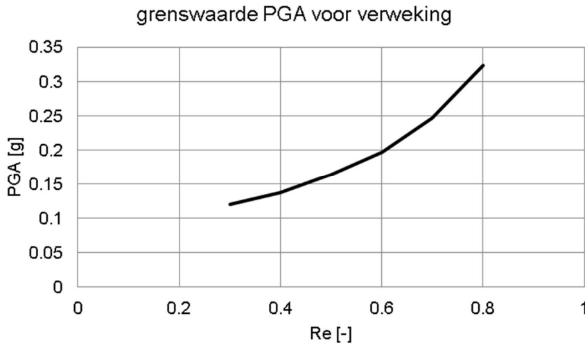
Figuur 6.6 Grenswaarden PGA bij verschillende relatieve dichtheden (Re) voor begin verweking
