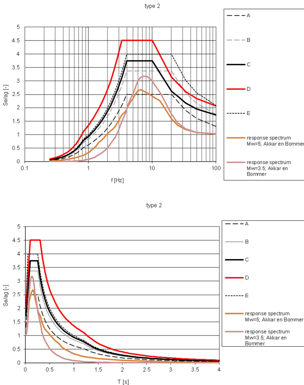
Figuur 4.6 Vergelijking van verschillende ontwerpspectra voor belasting (boven in frequentiedomein, onder in tijddomein)
