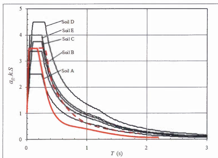
Figuur 2.1 Voorlopige inschatting van elastisch respons spectrum (bij \zeta = 5\% damping)
