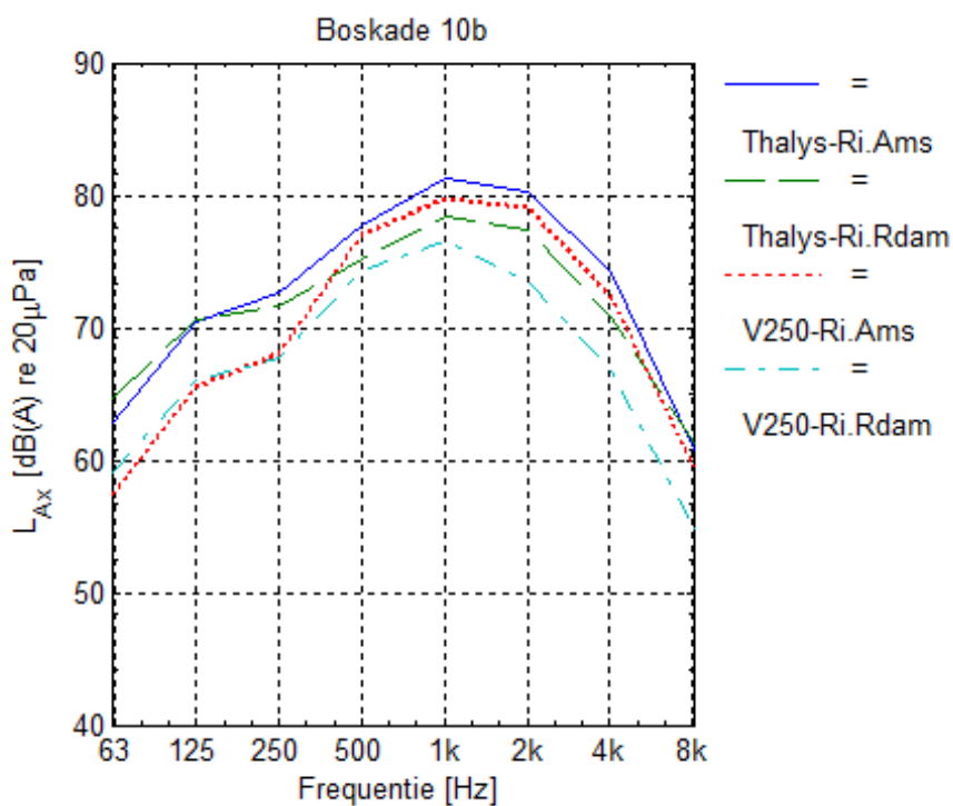
Figuur 7 Gemeten gemiddelde A-gewogen geluidexpositieniveaus L_{Ax} (dB(A) re. 20 \mu Pa), in octaafbanden, bij de woning aan de Boskade 10B, van alle geanalyseerde treinpassages van de Thalys en Ansaldo V250 per rijrichting.
