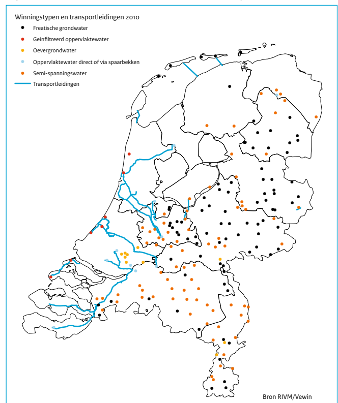
Figuur 2.1 Hoofdinfrastructuur drinkwatervoorziening
