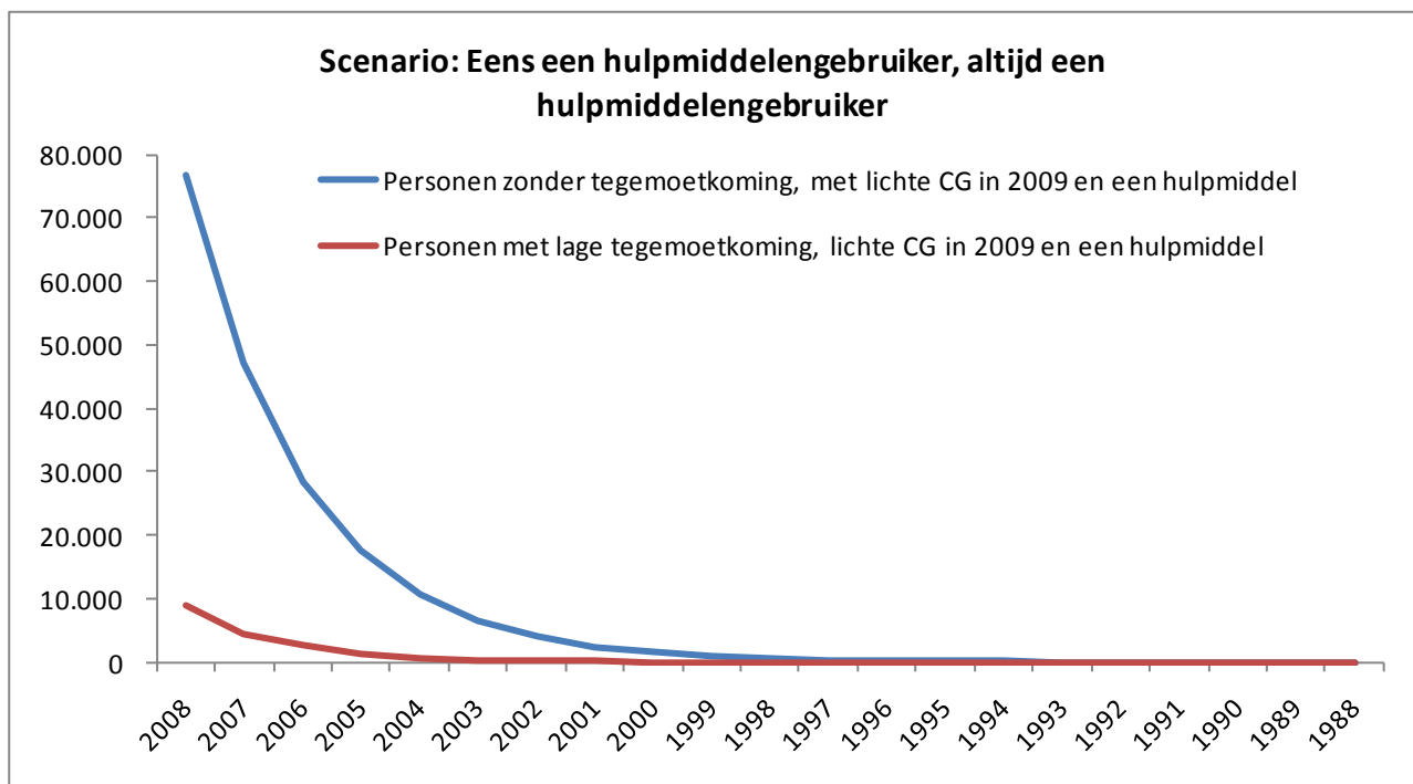
Figuur 3: Effect meerjarig hulpmiddelengebruik op de Wtcg wanneer uit wordt gegaan van de aanname dat iemand die eens een hulpmiddel gebruikt altijd een hulpmiddel gebruikt.
