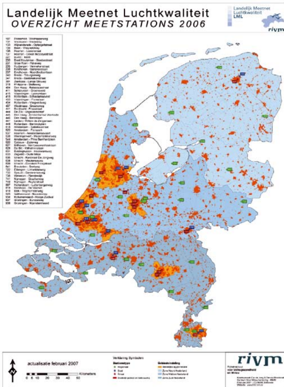
Figuur 1 Overzicht van Nederland met agglomeraten in oranje- en zones in blauwe schaduw aangegeven. In gekleurde boxen (groen: regionaal, blauw: stedelijk, rood: straat) zijn de stations van het Landelijk Meetnet Luchtqualiteit aangegeven.
