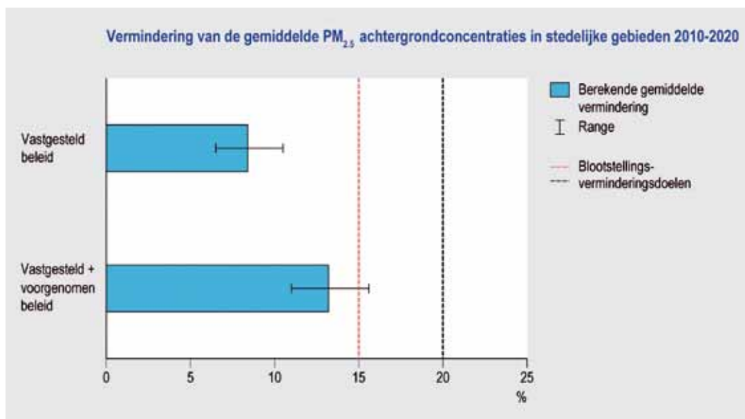
Figuur 0.3: Vermindering van de gemiddelde \text{PM}_{2.5} concentratie in stedelijke gebieden tussen 2010 en 2020
