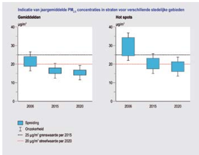
Figuur 0.2: Indicatie van de ontwikkeling van de gemiddelde PM_{2.5} concentratie in stedelijke gebieden tot 2020
